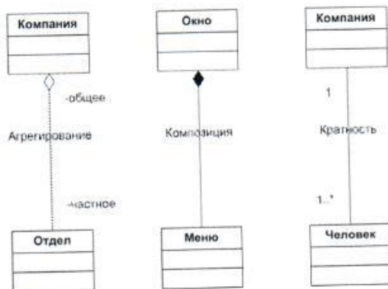
Рис. 13. Дополнения к отношению ассоциация на диаграмме классов
