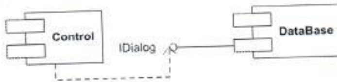
Рис. 17. Фрагмент диаграммы компонентов
