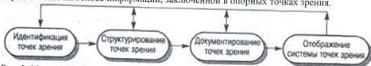
Рис. 3. Метод VORD
