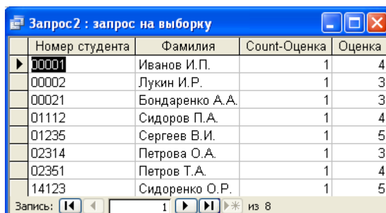
Рис. 20. Результаты запроса на группирование данных
